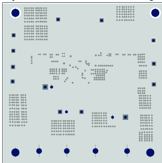
Figure 5—Bottom Layer
