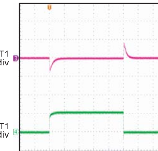
100 \mu s /div.
