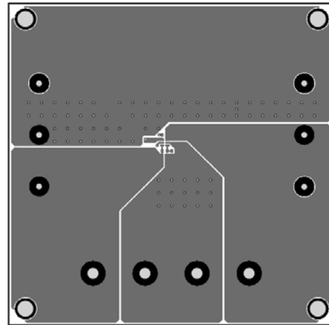
Figure 3—Top Layer
