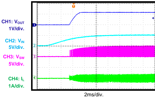
V_{IN} 上电 I_{OUT} = 0A
