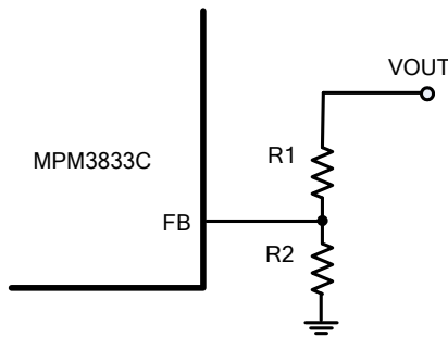
图 2: 反馈网络
