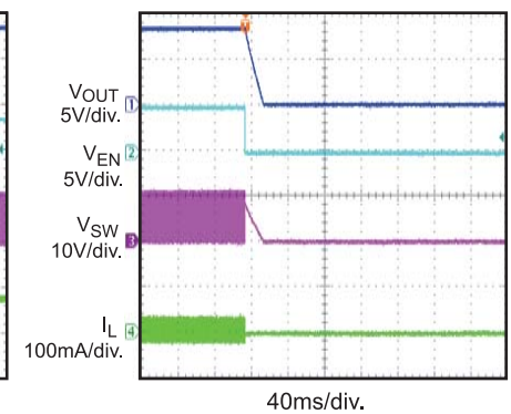
EN Shutdown
