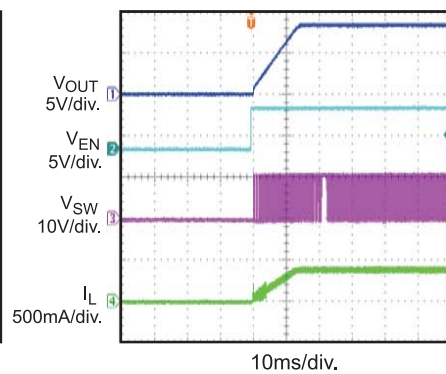
EN Start-Up
