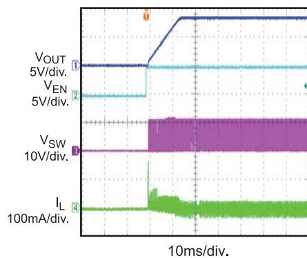
EN Start-Up
