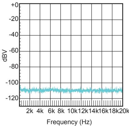
FFT Noise Floor Test (12V, 4Ω+33μH)
