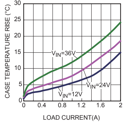
Thermal Rise
