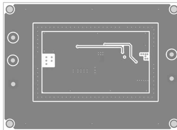
Figure 5—Bottom Layer
