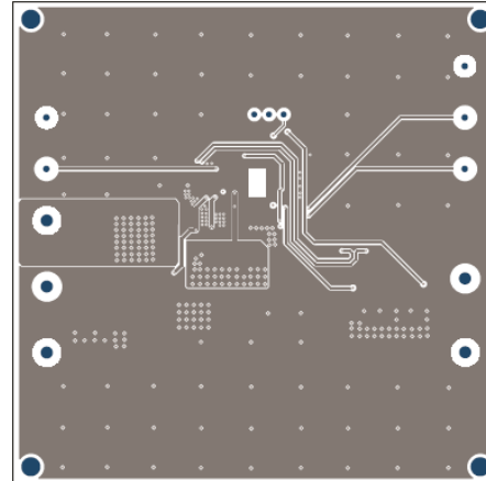
Figure 4— Middle Layer 2
