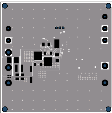
Figure 5—Bottom Layer
