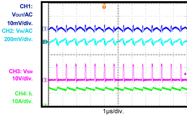
Input/Output Ripple
