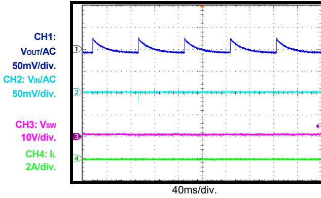
Input/Output Ripple
