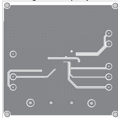
Figure 4— Inner Layer 2
