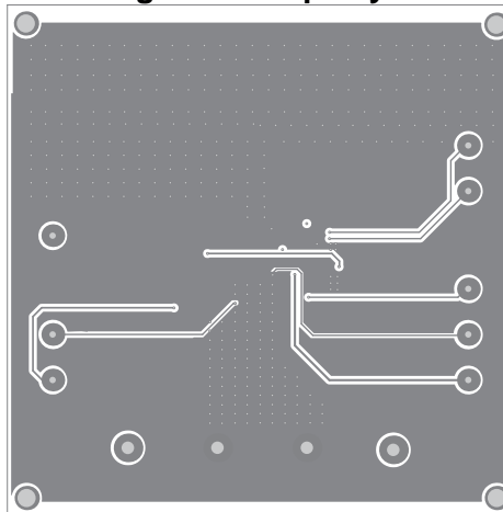
Figure 4— Inner Layer 2
