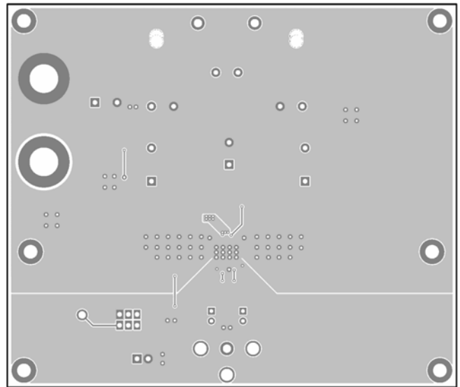
Figure 4—Bottom Layer
