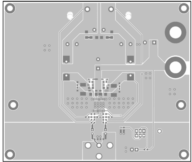
Figure 2—Top Layer
