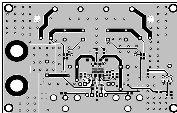
Figure 2—Top Layer
