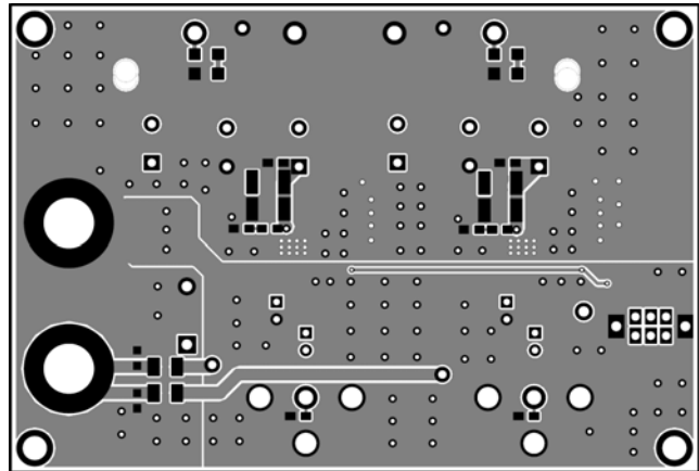
Figure 4—Bottom Layer
