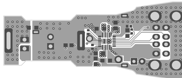
Figure 6—Bottom Layer
