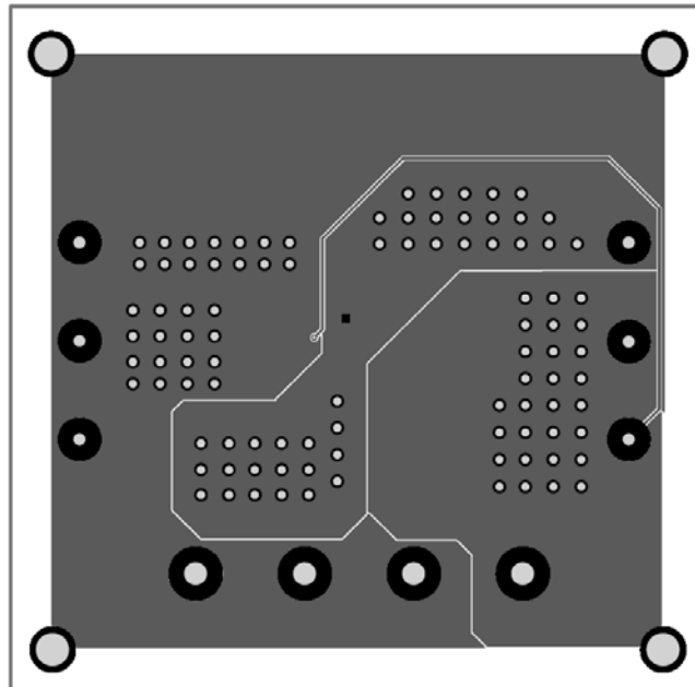
Figure3: Bottom Layer
