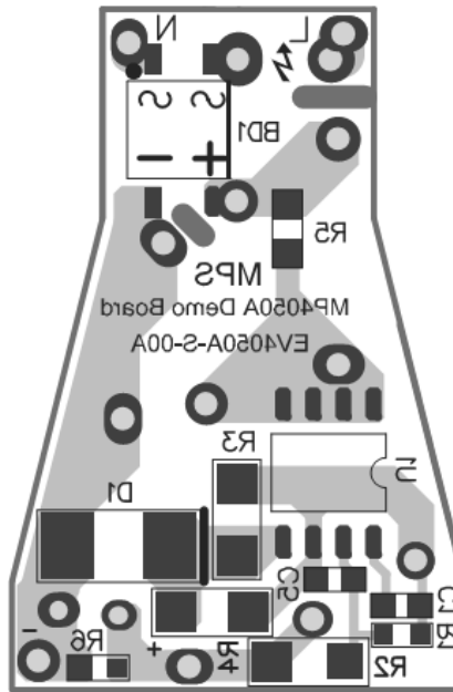
Figure 3—Bottom Layer
