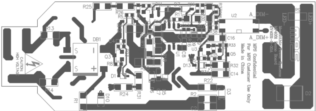
Figure 3—Bottom Layer
