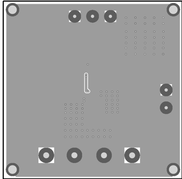
Figure 2—Bottom Layer
