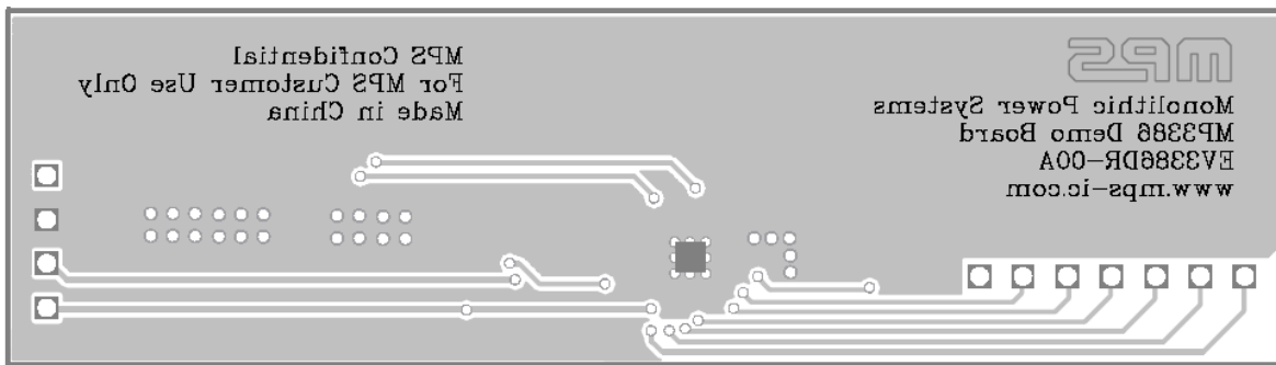
Figure 2—Bottom Layer
