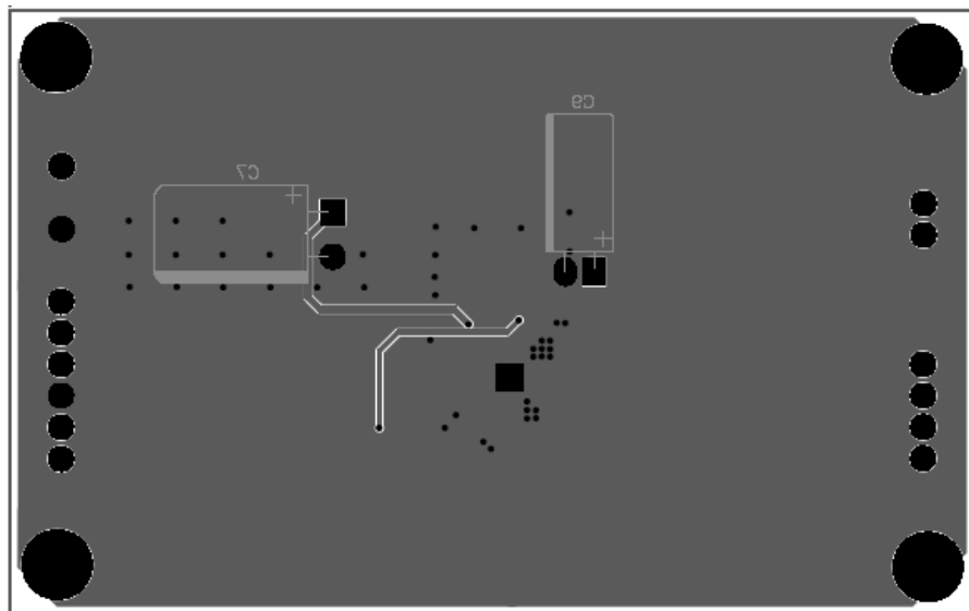
Figure 2—Bottom Layer
