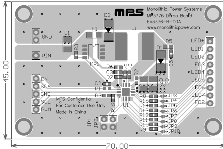
Figure 1—Top Layer
