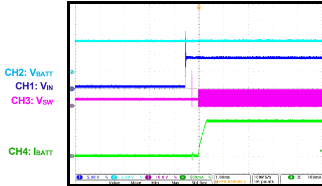
VIN Hot Plug-In
