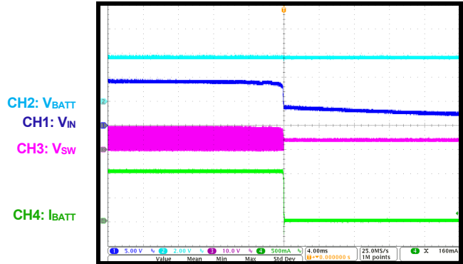
VIN Hot Plug-Out
