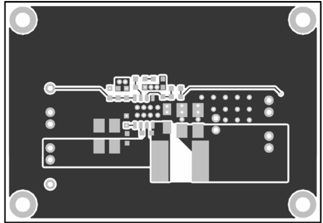
Figure 2—Top Layer
