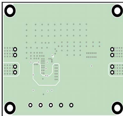
Figure 3—Bottom Layer
