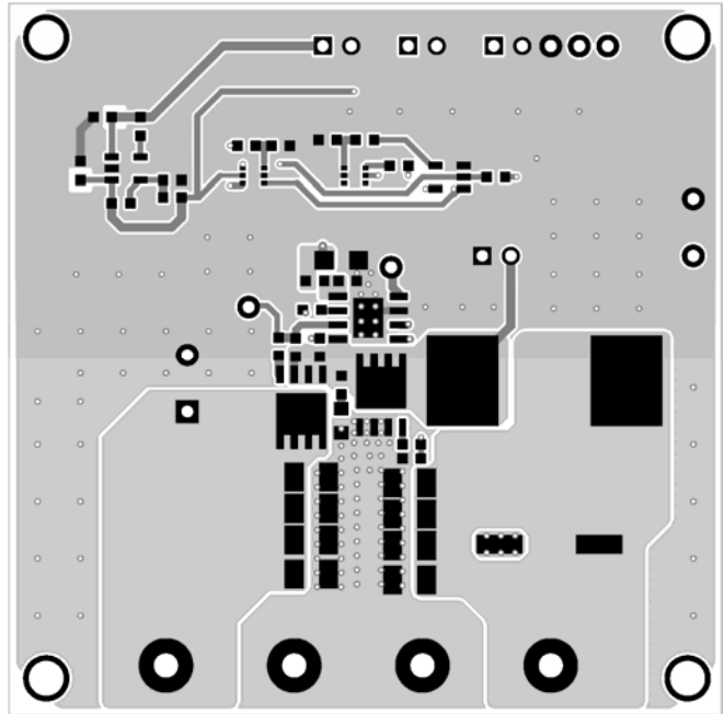
Figure 2—Top Layer
