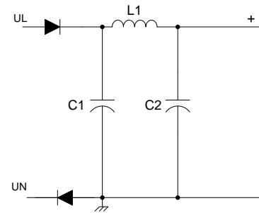
图 10: 半波整流器
