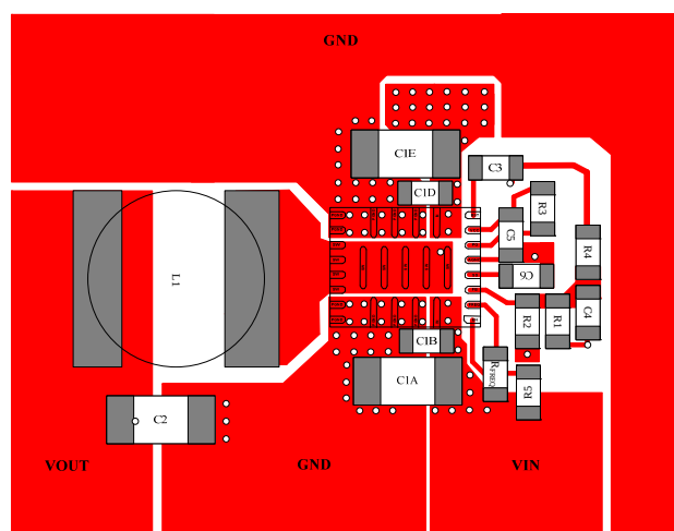
Top Layer
