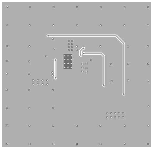
Inner 2 Layer
