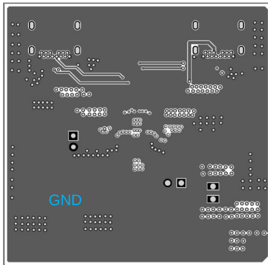
Middle Layer 2
