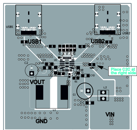
Top Layer
