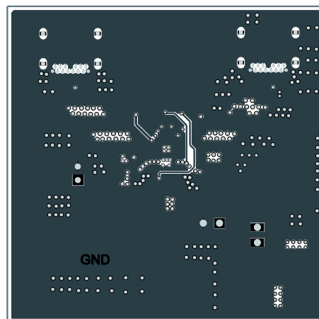
Middle Layer 2
