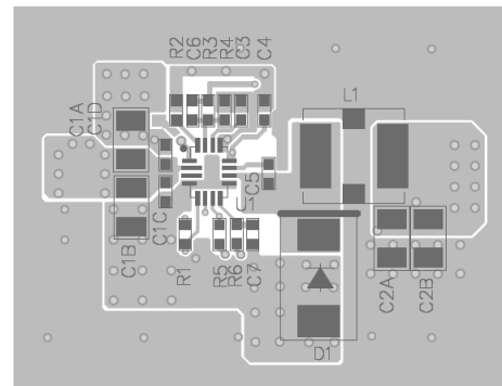
Top Layer
