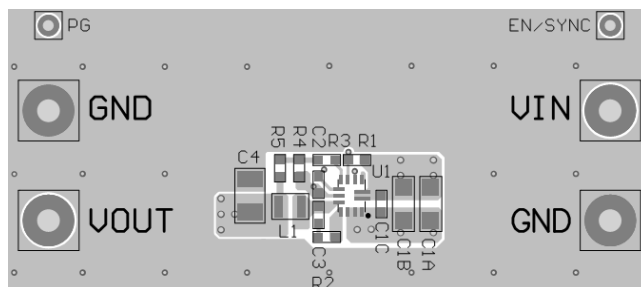
Top Layer
