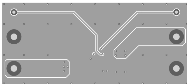
Inner Layer 2
