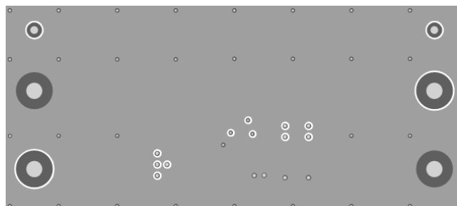
Inner Layer 1
