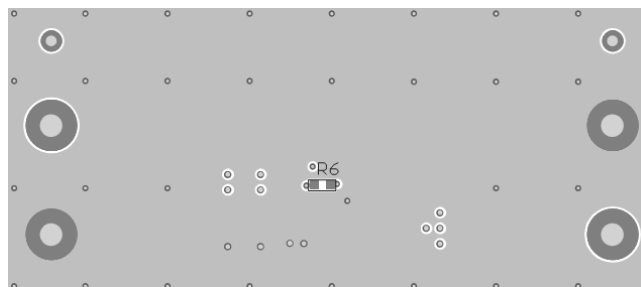
Bottom Layer
