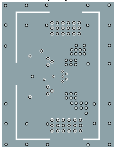
Inner Layer 1
