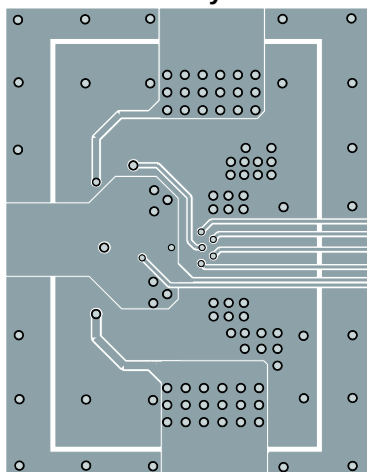
Inner Layer 2
