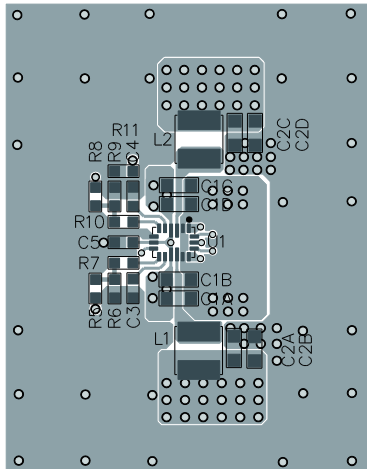
Top Layer
