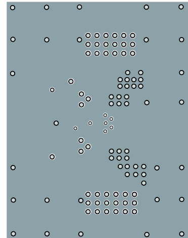
Bottom Layer
