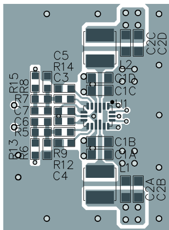
Top Layer
