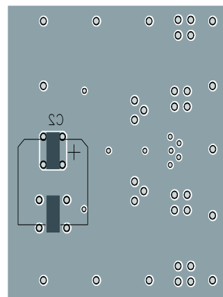
Bottom Layer
