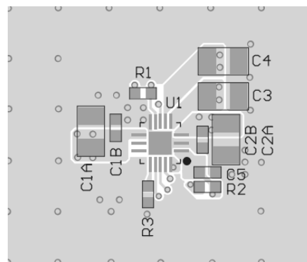
Top Layer
