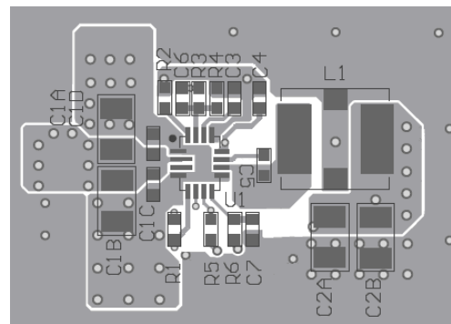
Top Layer
