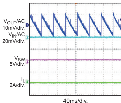
Input/Output Ripple
