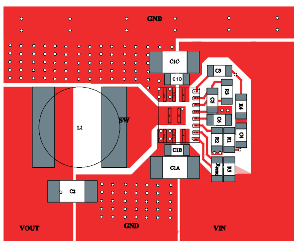
Top Layer
