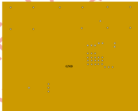
Inner1 Layer
