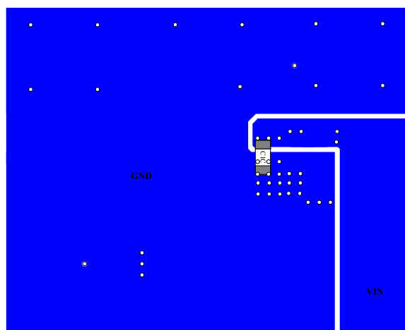
Bottom Layer
