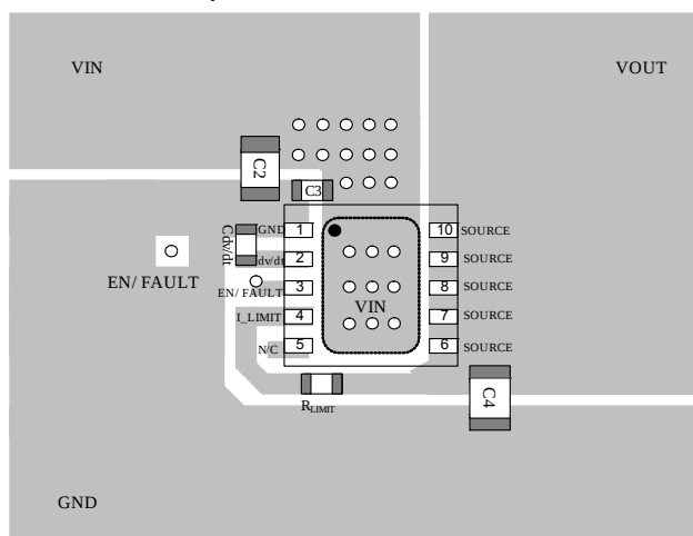
Top Layer
