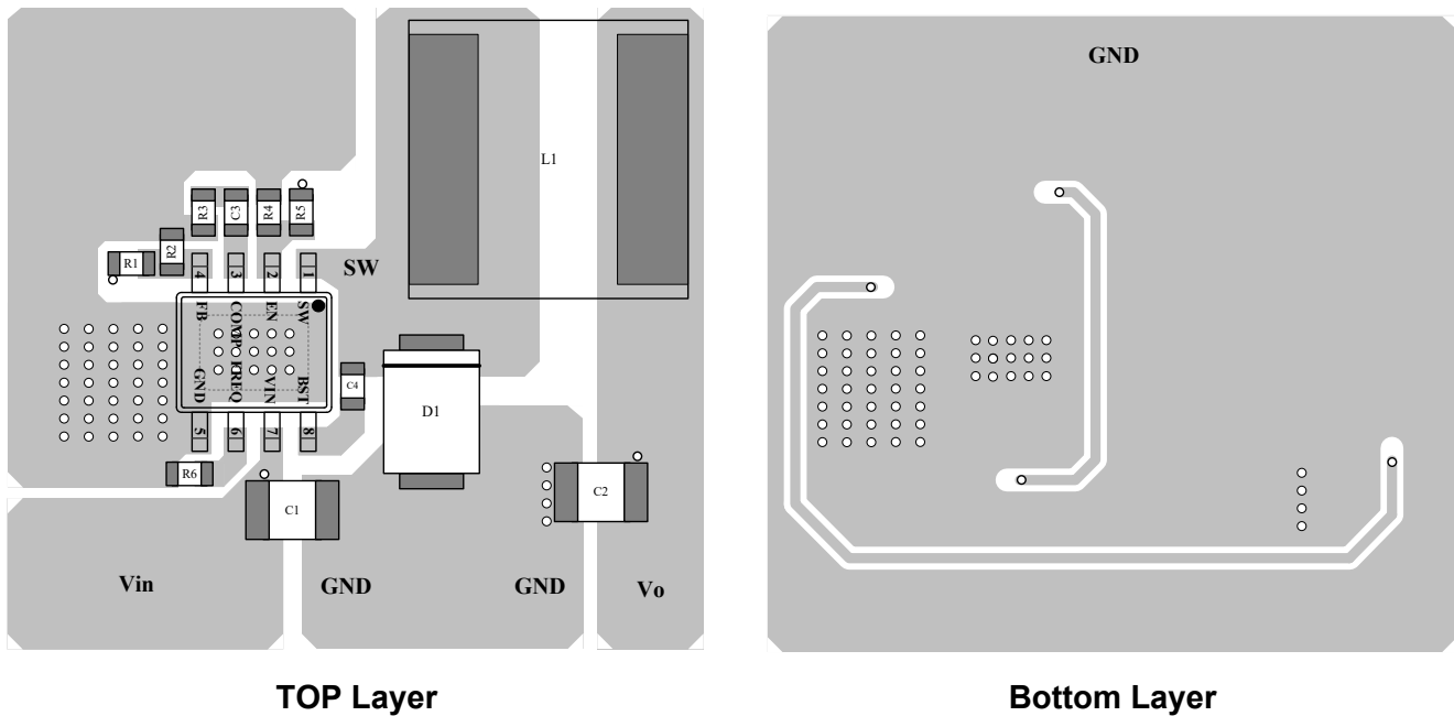
MP4560DN Layout Guide
