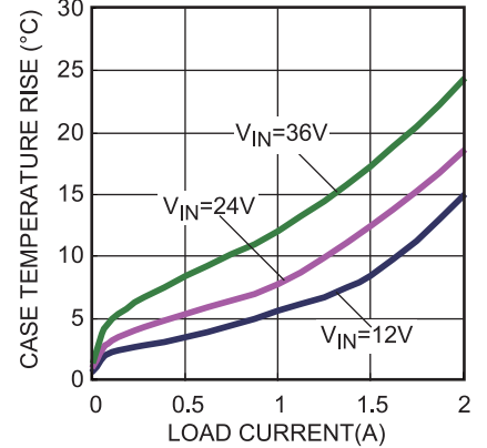
Thermal Rise
