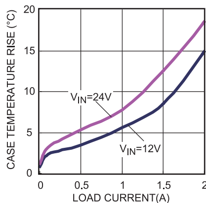
Thermal Rise
