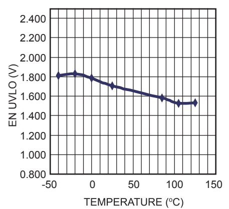
EN UVLO vs. Temperature
