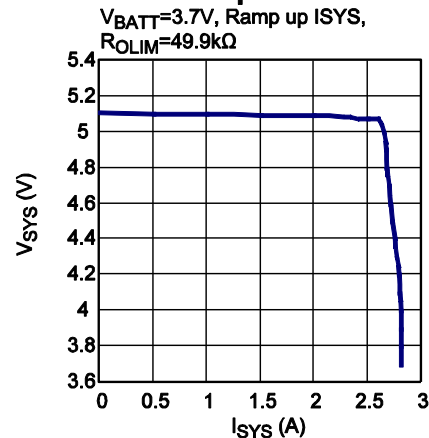
Boost Output U-I
