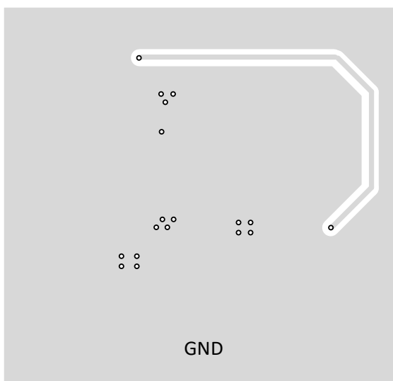
Bottom Layer
