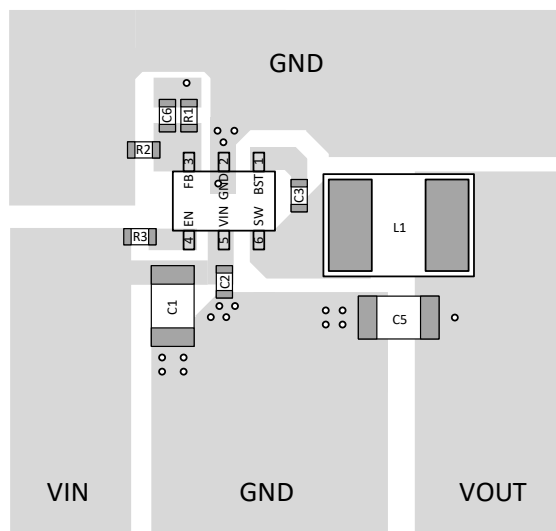
Top Layer
