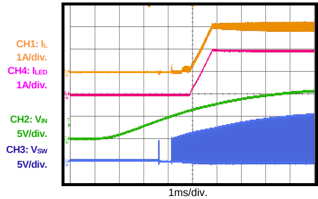
VIN Start-Up
