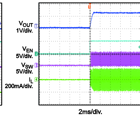
EN Start-Up
