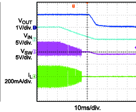
VIN Shutdown
